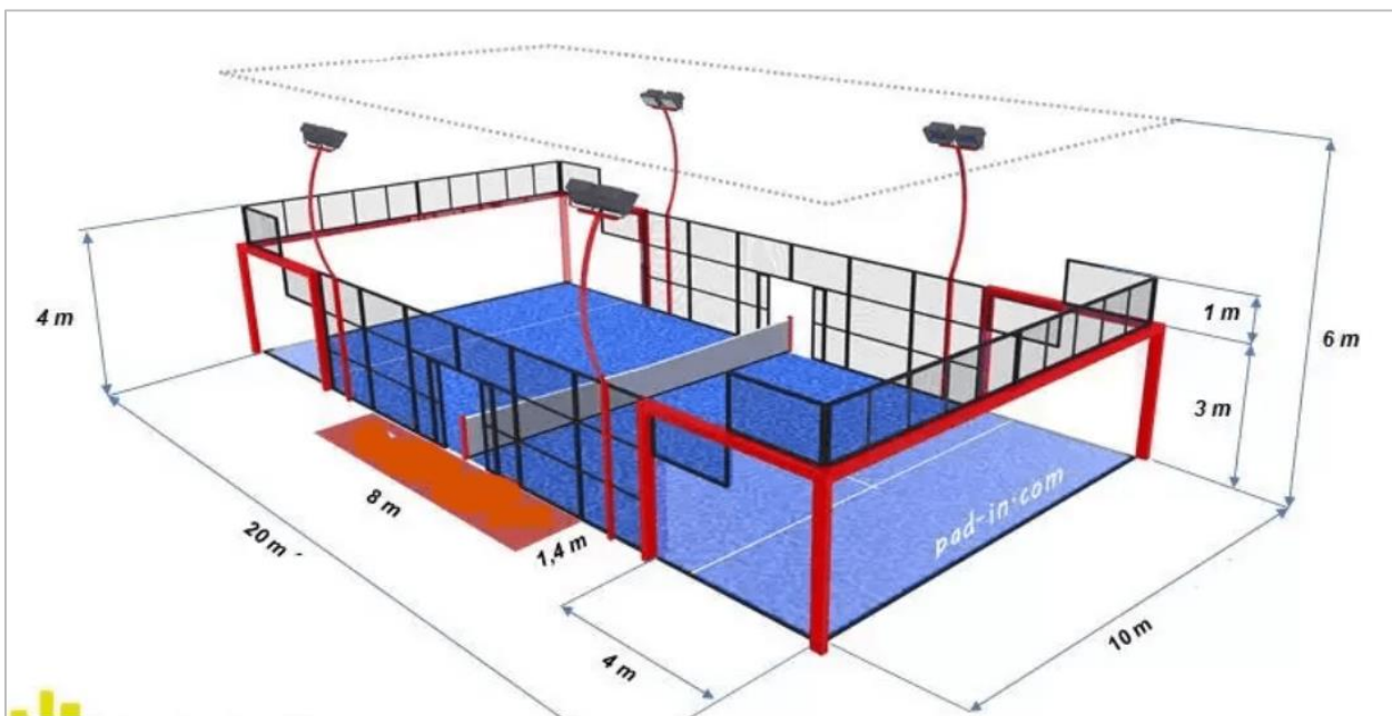
Figure 4 Schéma des dimensions d'un terrain de padel
