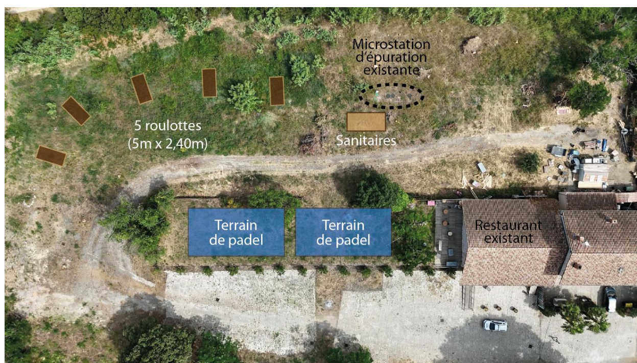
Figure 7 : Emplacement des installations et des terrains de padel du STECAL à Cruzy
